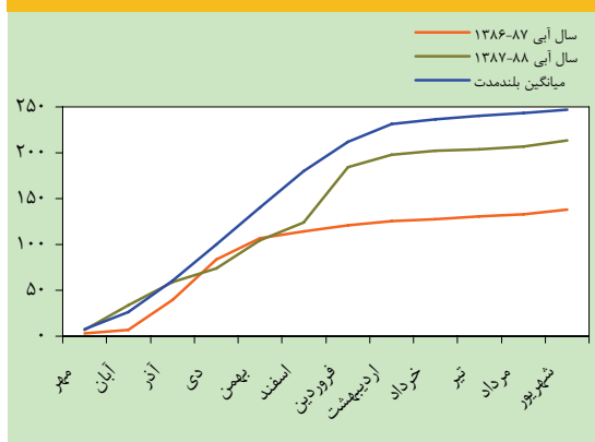
نمودار ۳-۱- ارتفاع تجمعی بارندگی (میلی‌متر)
